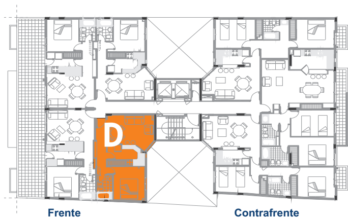
PLANTA DEL EDIFICIO
