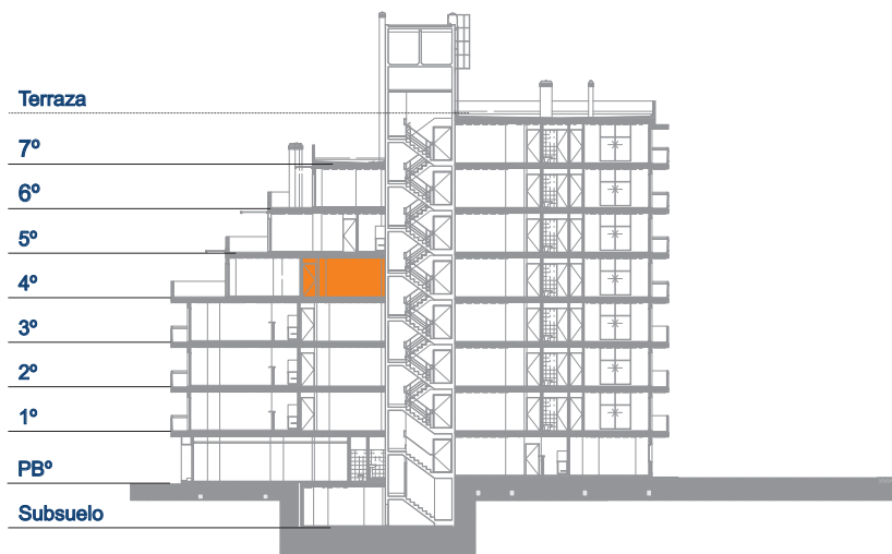
CORTE DEL EDIFICIO
